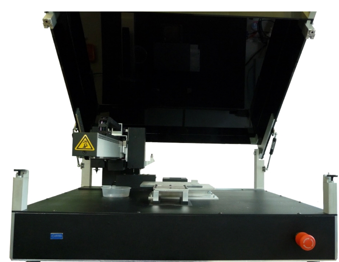
Automatischer Aufbau (Pick-and-Placer)
